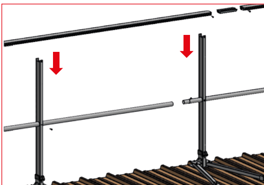
7 - Clipser la main courante dans les montants. Fixez la avec la vis autoforeuse 4,8x16. Couple de serrage recommandé 5 N.m.
