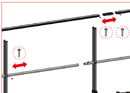
9 - Assembler les mains courantes avec les jonctions et les sous-lisses des tronçons montés. Fixer chaque jonction avec les vis 4,8 x 16 : 2 à chaque jonction de main courante et 1 entre 2 sous-lisse.
