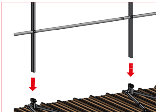
5 - Placer le tout dans les embases.
