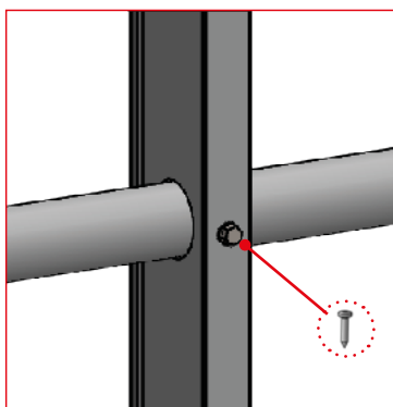
8 - Visser les vis 4,8 x 32 sur le montant au niveau de la sous-lisse.
