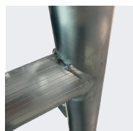
Structure en aluminium soudé, montants de 50mm
