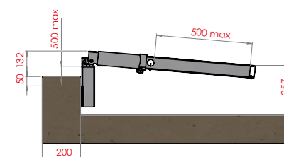
Applique déporté 130 mm
