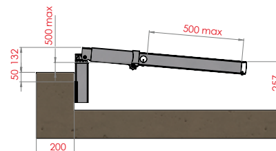
Applique déporté 110 mm
